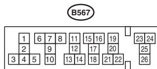
继电器支架
